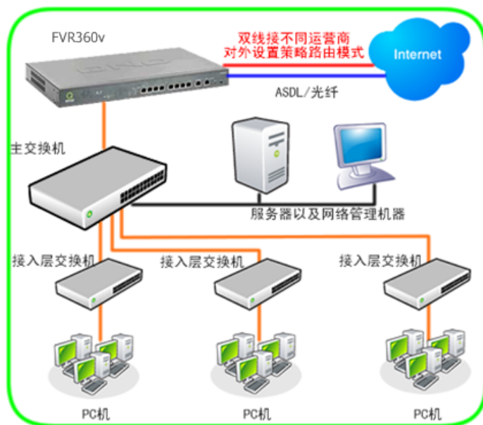
图：FVR360v 双线不同运营商 ADSL/光纤连入互联网
