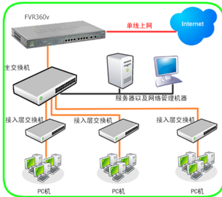
图：FVR360v 单线 ADSL/光纤连入互联网
