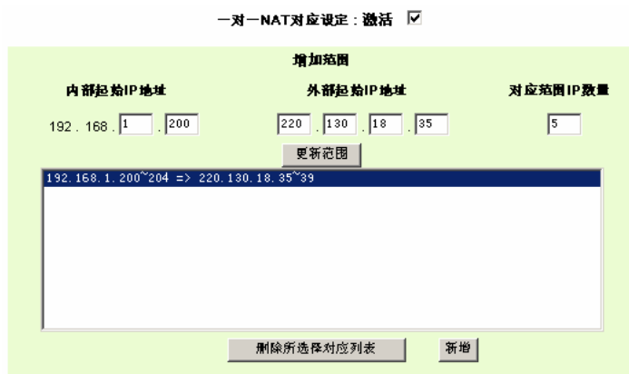
图：一对一 NAT 配置画面
