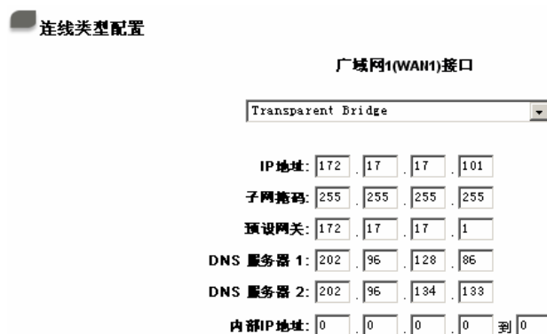
图：通透桥接模式 的配置画面
