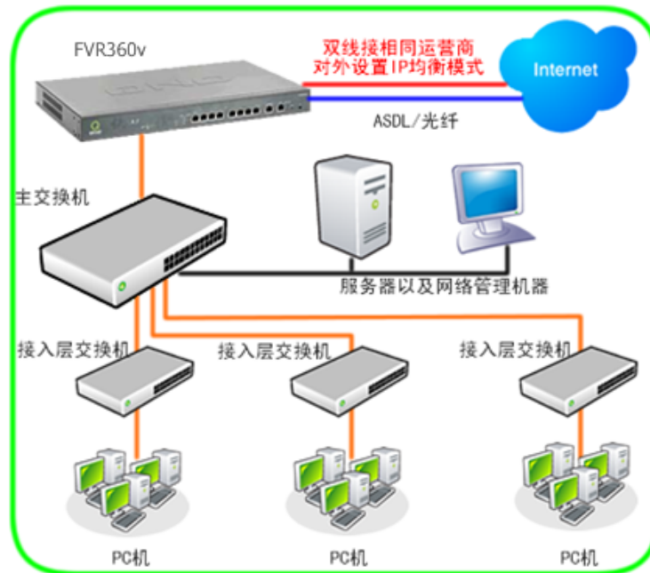
图：FVR360v 双线相同运营商 ADSL/光纤连入互联网
